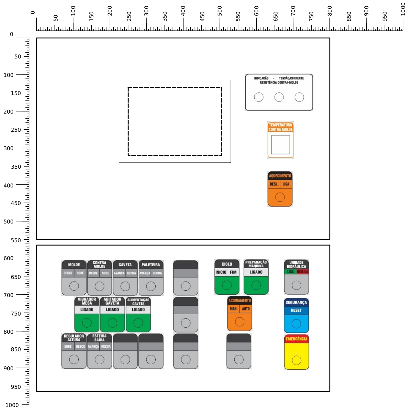
LAYOUT MESA DE COMANDO
