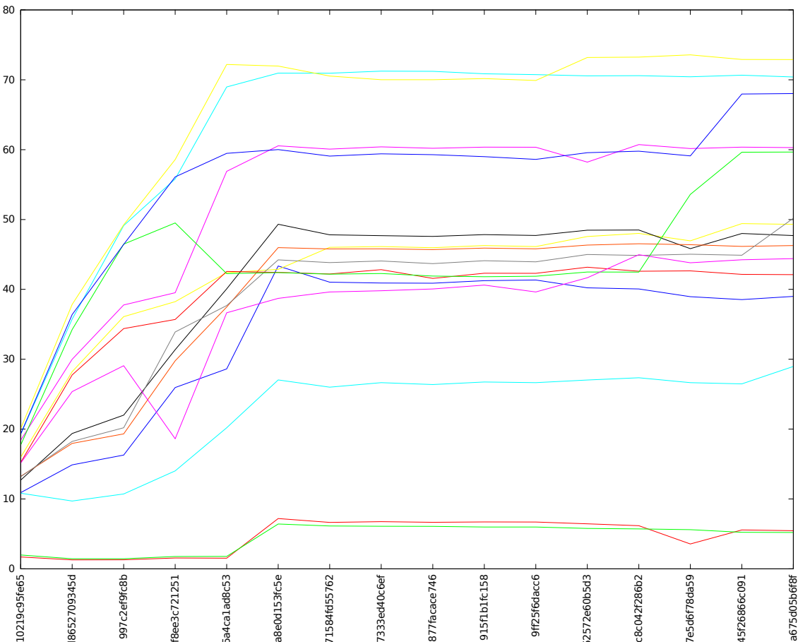
haswell-fma-sgemmm
